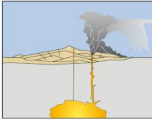
1. Eruption aus einem (Seiten-)Krater
