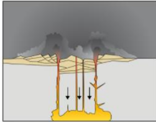
2. Der Boden senkt sich durch die einstürzende Magmakammer
