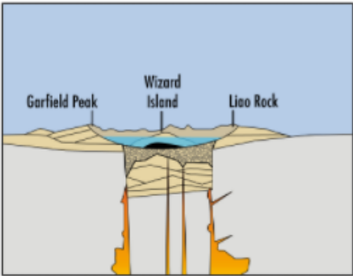
4. Die erkaltete Caldera füllt sich mit einem Calderasee
