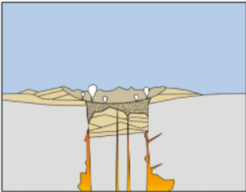
3. Asche- und Geröllablagerungen am Boden; eindringendes Grundwasser kann zu Geysiren führen
